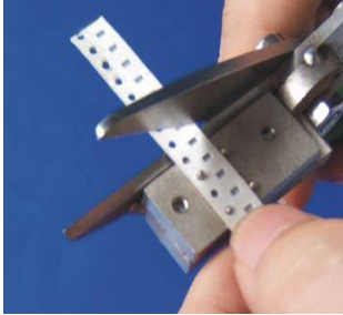
1、将料带放在专用剪刀上，沿孔的中心剪齐
