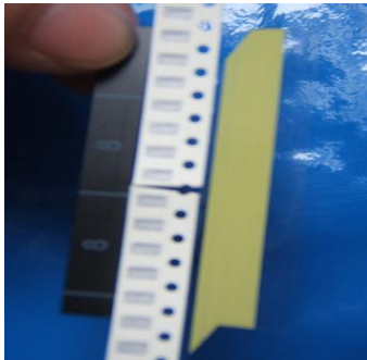
1、将料带放在专用剪刀上，沿孔的中心剪齐
